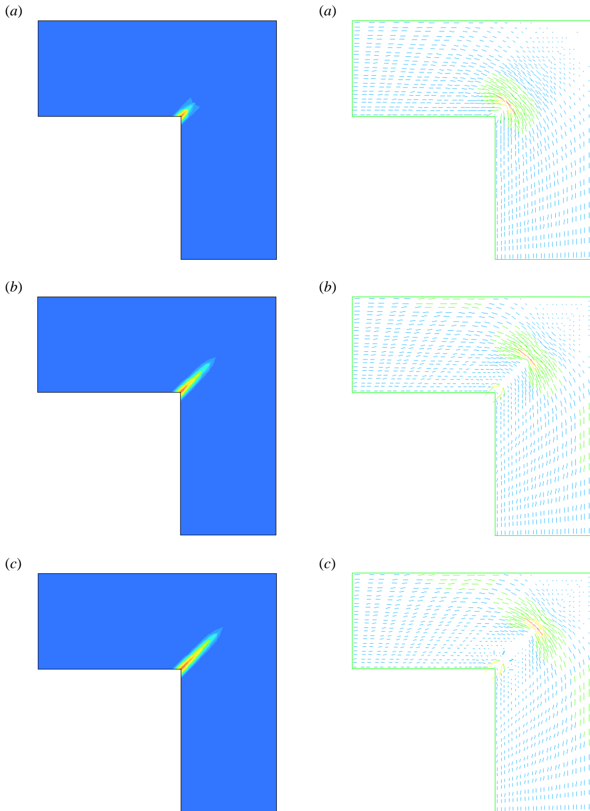
Figur 17 Spröd puts, töjnings- och spänningsfördelning. (a) krympning = 0.024 mm/m, (b) krympning = 0.032 mm/m, (c) krympning = 0.040 mm/m.
