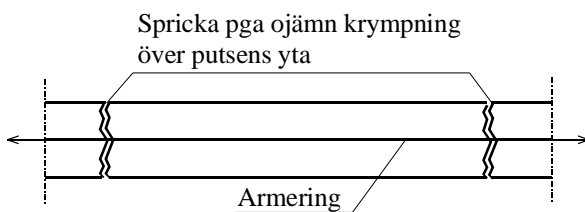
g) Jämn krympning genom tvärsnittet och ojämna krympning över putsytan, rak armering.
