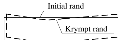
f) Ojämn krympning genom tvärsnittet och över ytan
