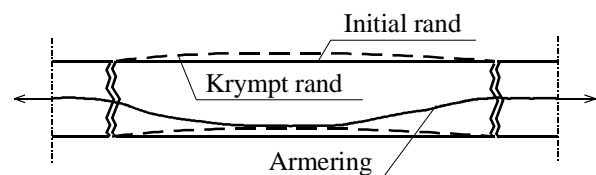
h) Jämn krympning genom tvärsnittet och ojämna krympning över putsytan, böjd armering.
